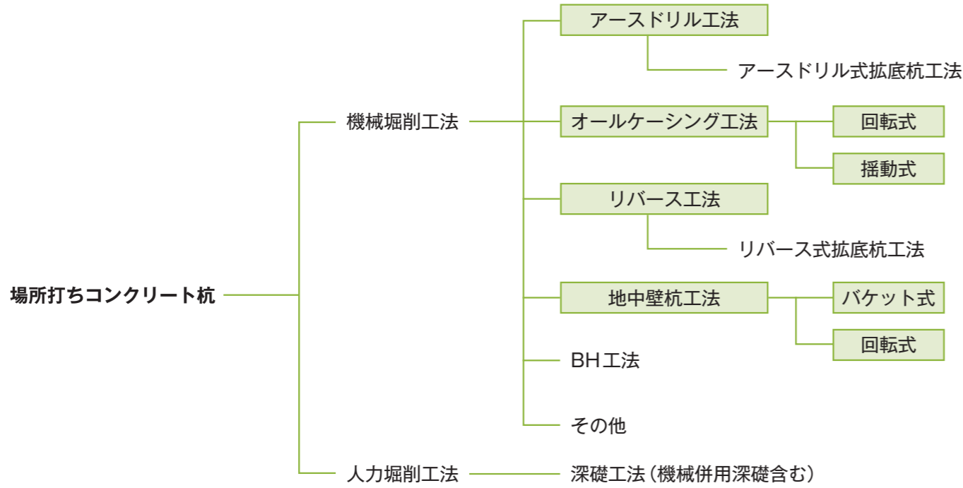
場所打ちコンクリート杭の施工法による分類
